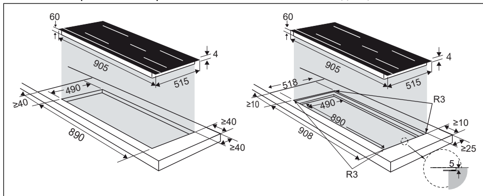
Установка на рабочей поверхности
